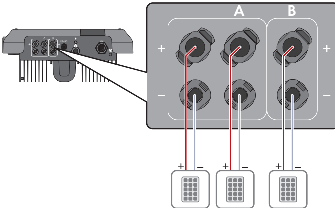
Figura 10: Panoramica del collegamento nel funzionamento normale
